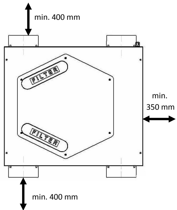
HRV 20 Deckenmontage
